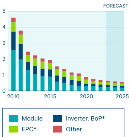
Solar PV capex benchmark 2022 $/W(DC)
